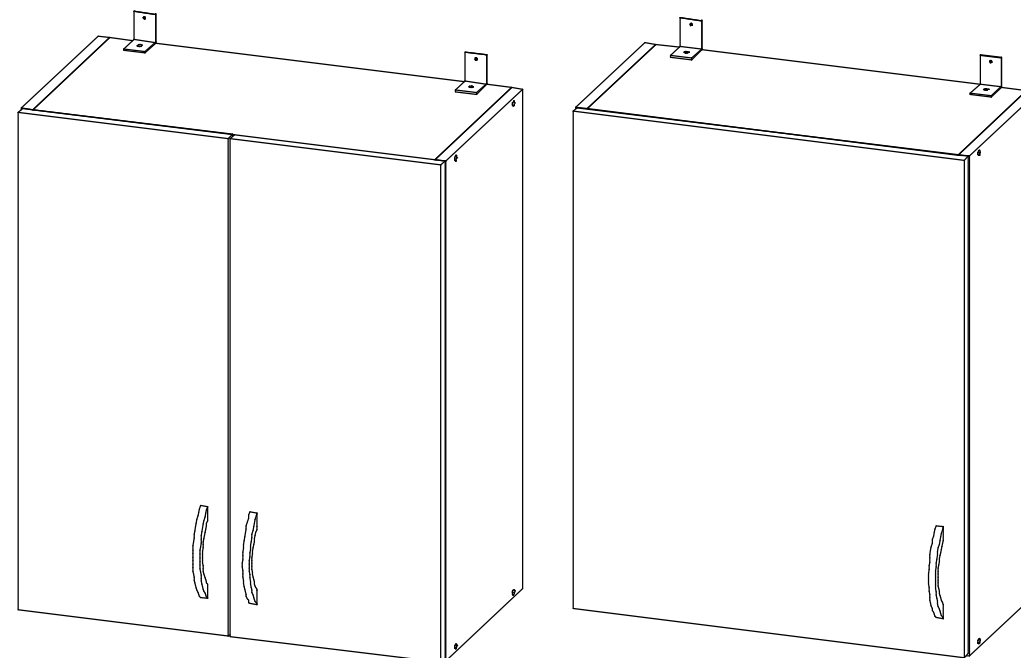
БИОЛА НЕО каркас Ш-600_Н9
